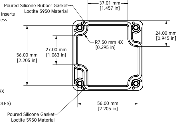
LID - INSIDE
