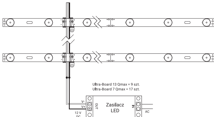
Rys. 1. Schematy prawidłowego podłączenia produktu do zasilacza.
